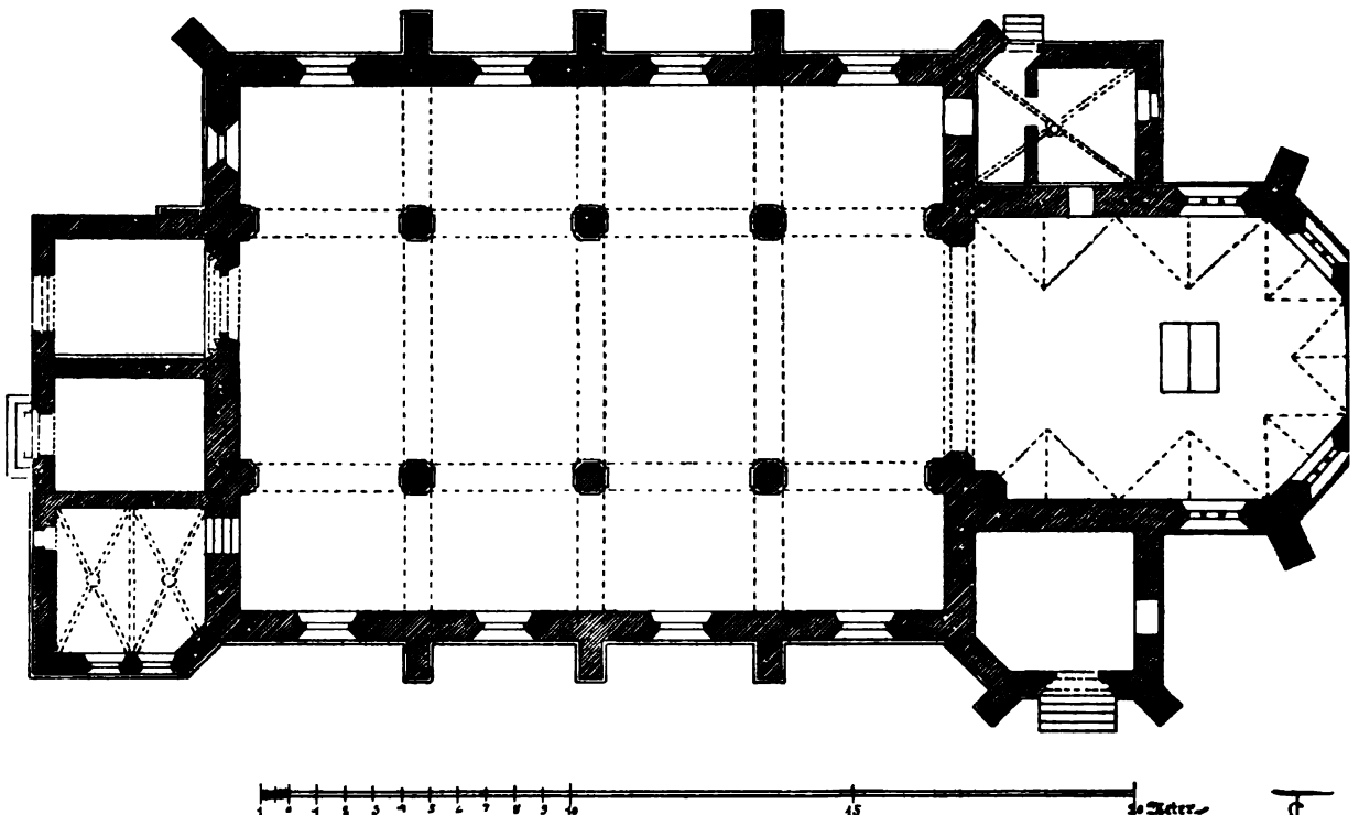
Grundriss der Kirche zu Schmölln.
